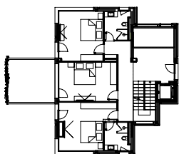
Първи етаж
